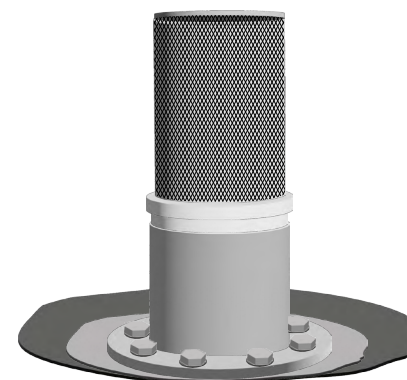
Vidange par le fond Bloc bride INOX boulonné Crépine INOX Manchon PVC-P 110 x 4" (raccordement tuyauterie enterrée à coller)
