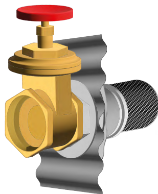
Vidange par le côté Vanne guillotine laiton DN100 Traversée de cloison INOX Crépine INOX
