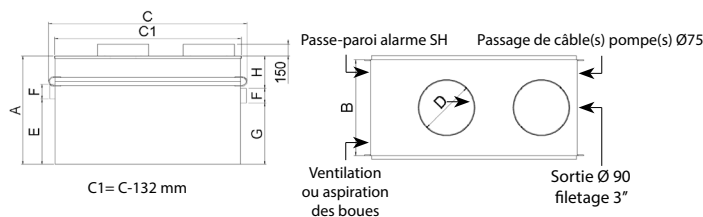
Séparateur d'hydrocarbures avec amorces circulaires :
