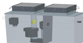
Séparateur d'hydrocarbures sans kit de fermeture
