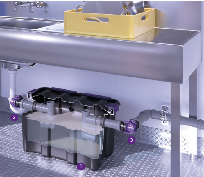
1 Séparateurs à graisses 2 Arrivée 3 Sortie
