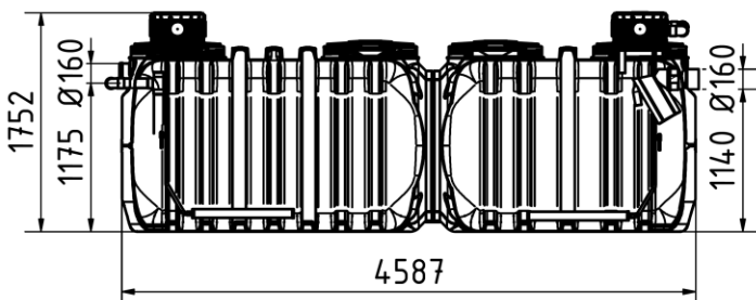
A-A ( 1 : 40 )
